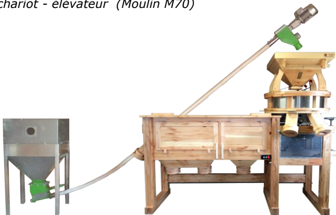
Exemple d'installation d'une trémie 750 litres avec vis de transport attenante + option de transport par chariot - élévateur (Moulin M70)
